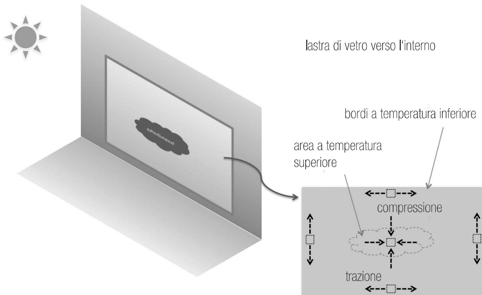
Figura 6. Carichi di origine termica generati in una vetrata esposta al riscaldamento da parte della radiazione solare; la pellicola applicata sulla superficie esterna di colore scuro causa un surriscaldamento localizzato del vetro
