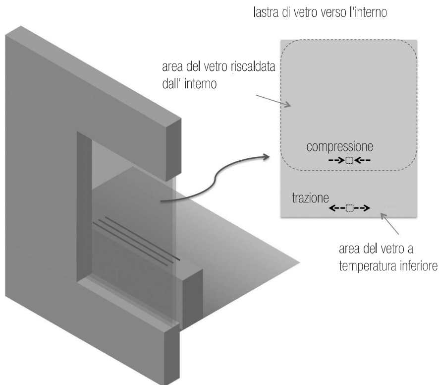
Figura 5. Carichi di origine termica generati nella lastra interna di una vetrocamera a causa della presenza di un ventilconvettore posizionato nelle immediate vicinanze del vetro e che lo riscalda non omogeneamente.
