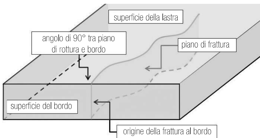
Figura 2: Conformazione della rottura per sbalzo termico
